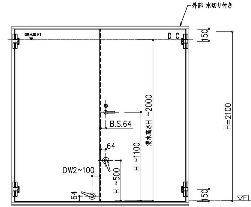
外観図
