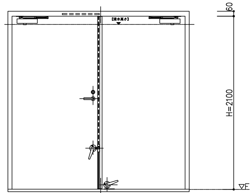
内観図
