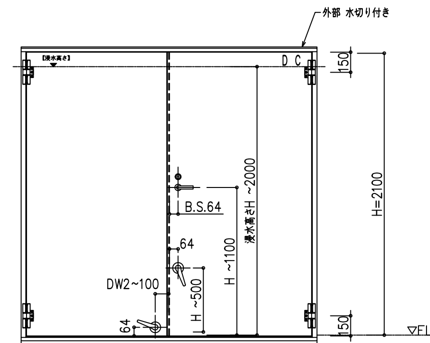
外観図
