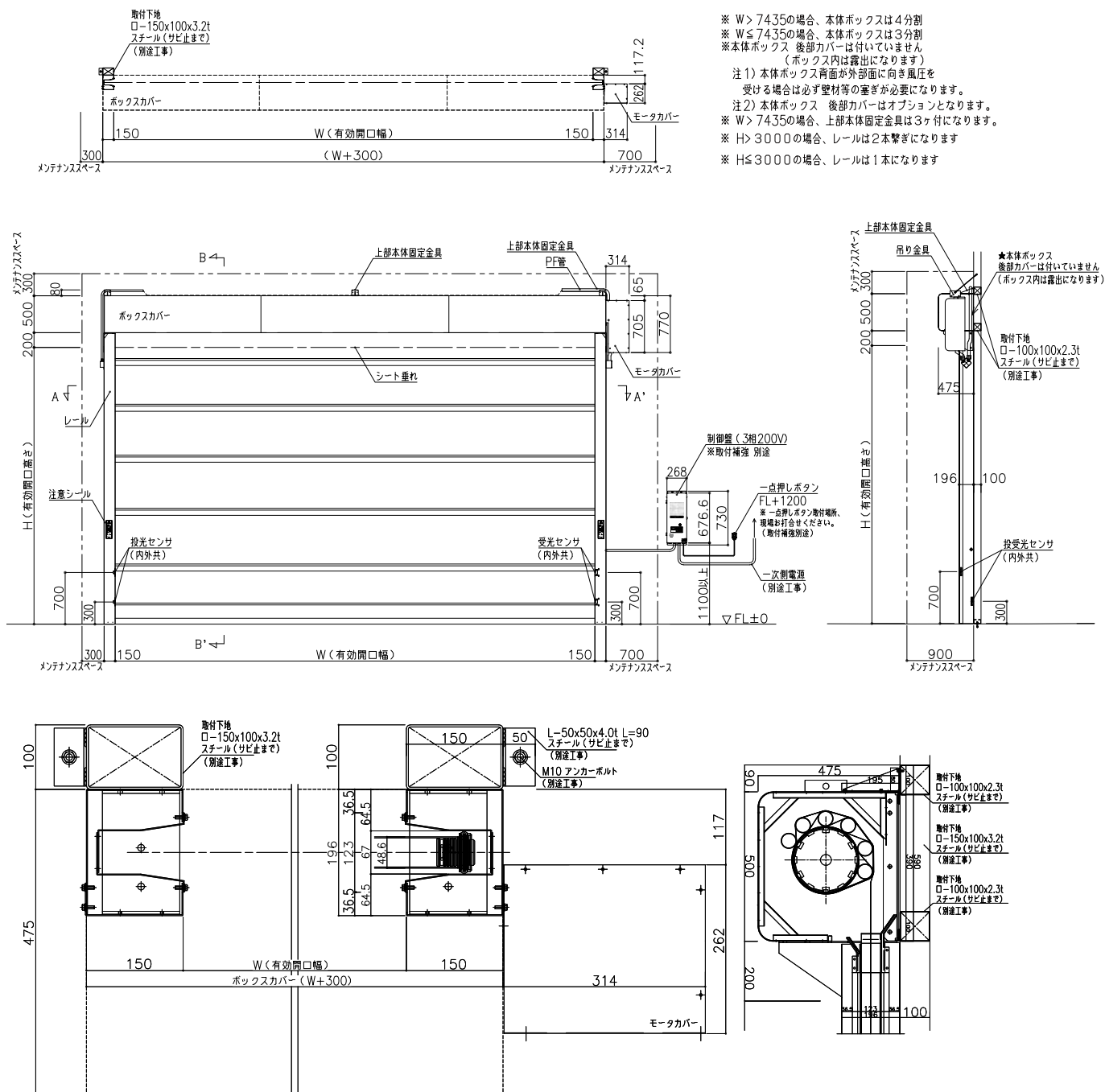
RX-4 納まり図
